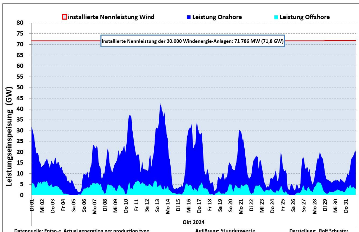
Abb. 1: Leistungsganglinie der Onshore/Offshore-Windenergie-Anlagen im Oktober 2024
