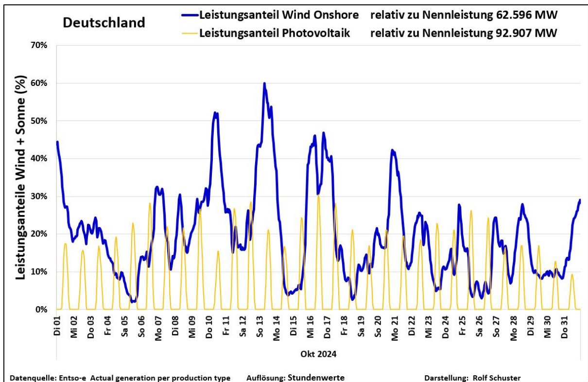
Abb. 5: Prozentuale Anteile EE Wind (Onshore) und Solar an der Leistungserzeugung im Okt. 2024
