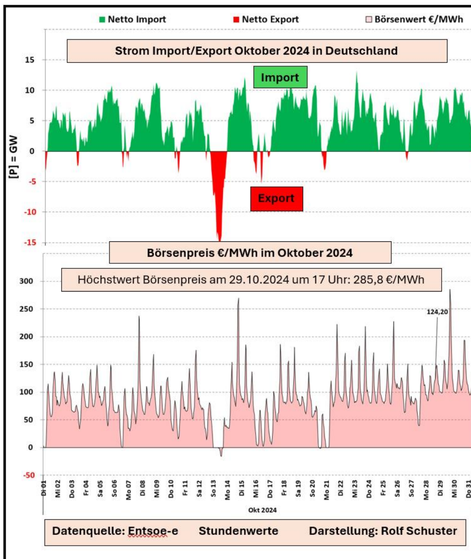
Abb. 7: Strom-Export/Import und Börsenentwicklung
