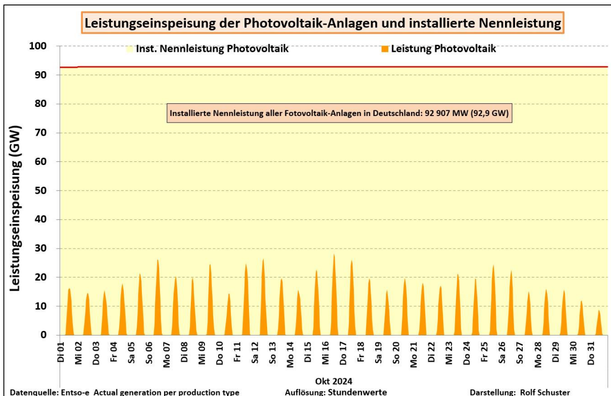
Abb. 2: Leistungsganglinie der Photovoltaik-Anlagen in Deutschland im Oktober 2024
